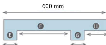
Vista Lateral
